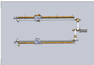
Y向双丝杆传动
