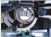
普通平缝机 Ordinary sewing machine
